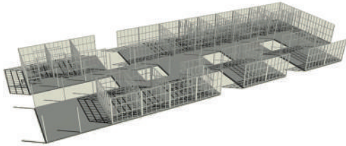
1. Cimentación y montantes
